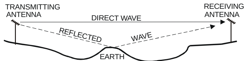
Figure 2-6. VHF LOS.
