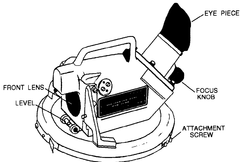
Figure 2-19. Telescopic alidade.
