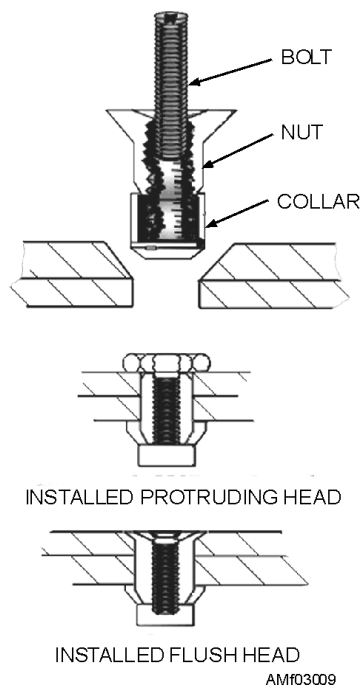
Figure 3-9.—Jo-bolt.
