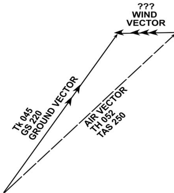
Figure 4.6-3 Actual Winds
