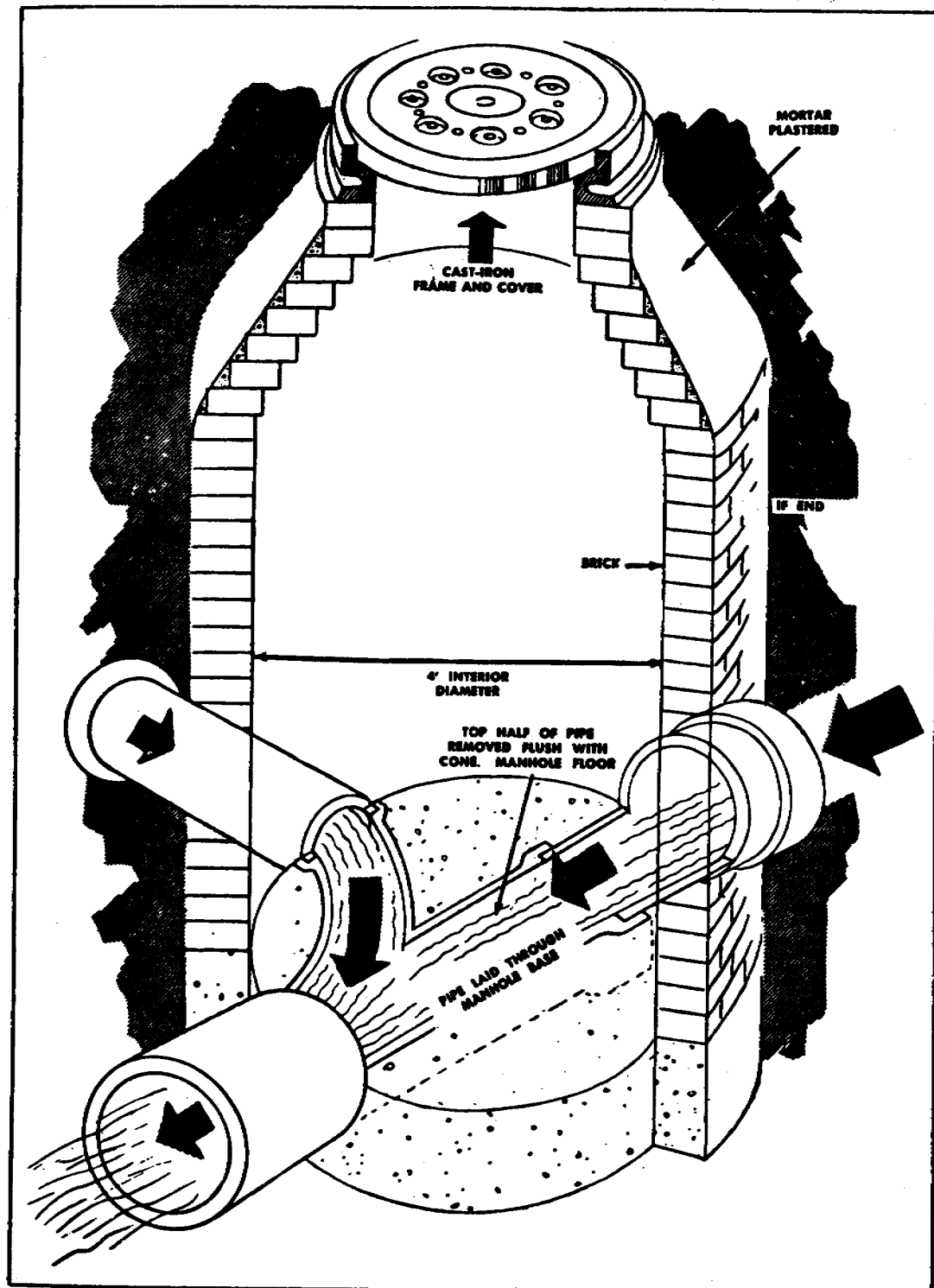
Figure 1-6. Manhole.
