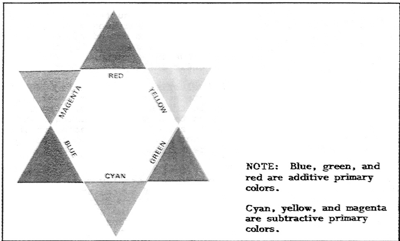
Figure 1-8. Color star
